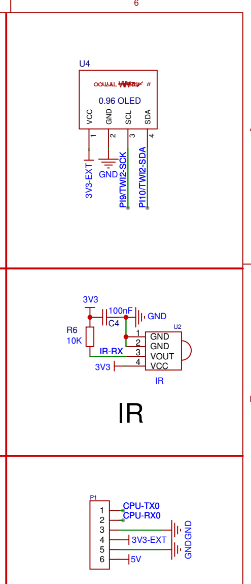
Debug
